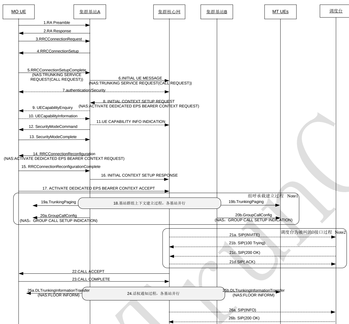
图9 单核心网下用户发起的组呼建立流程
